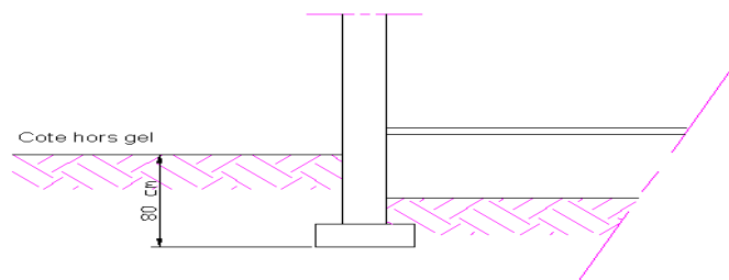
Profondeur d'ancrage des fondations
