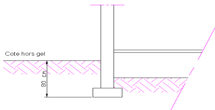
Profondeur d'ancrage des fondations
