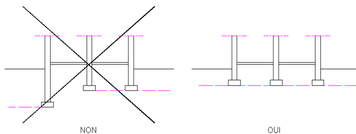
Plan d'assise des fondations
