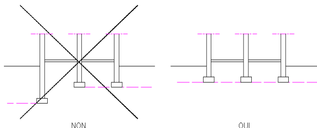
Plan d'assise des fondations
